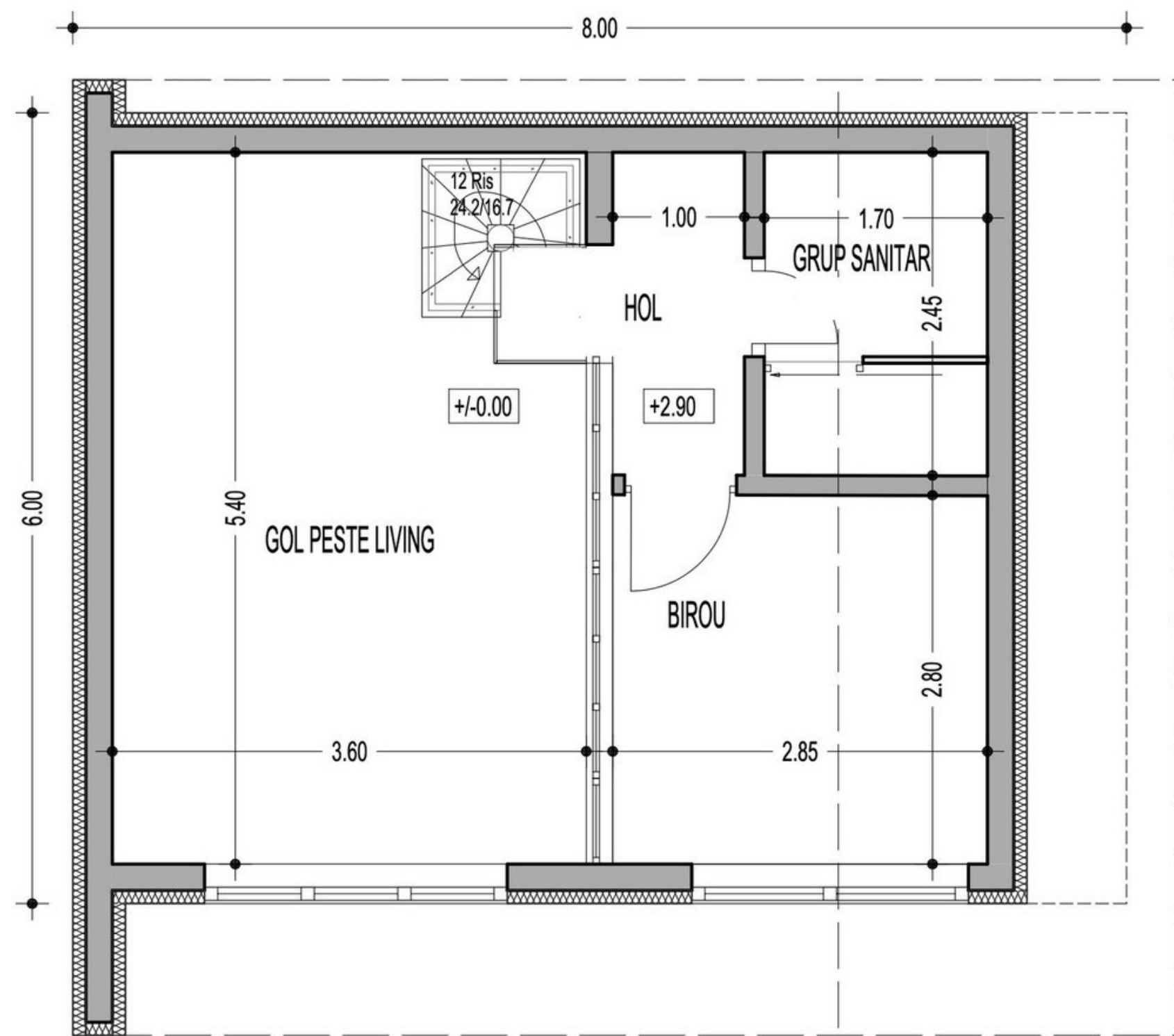
Loft Escape- Plan parter + etaj
